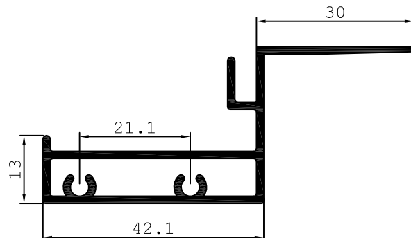
1022 0.674 Kg/M
