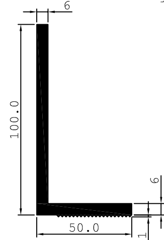
1020 FLUITED ANGLE 2.386 Kg/M
