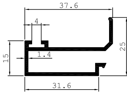
1017 CLIP 0.401 Kg/M
